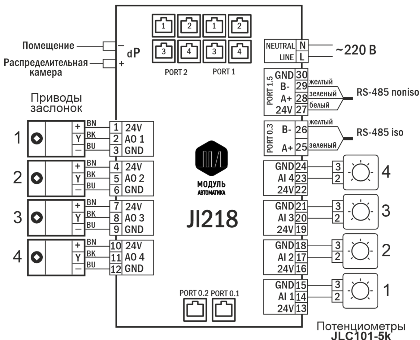
Рисунок 3.1 – Типовая схема включения
