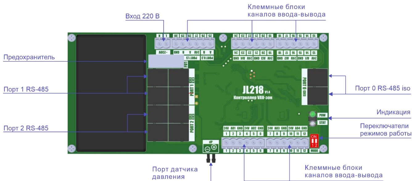
Рисунок 1.3 – Расположение элементов на плате контроллера
